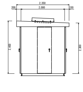
側面図 S=1/50 (姿図・寸法は参考とする)
