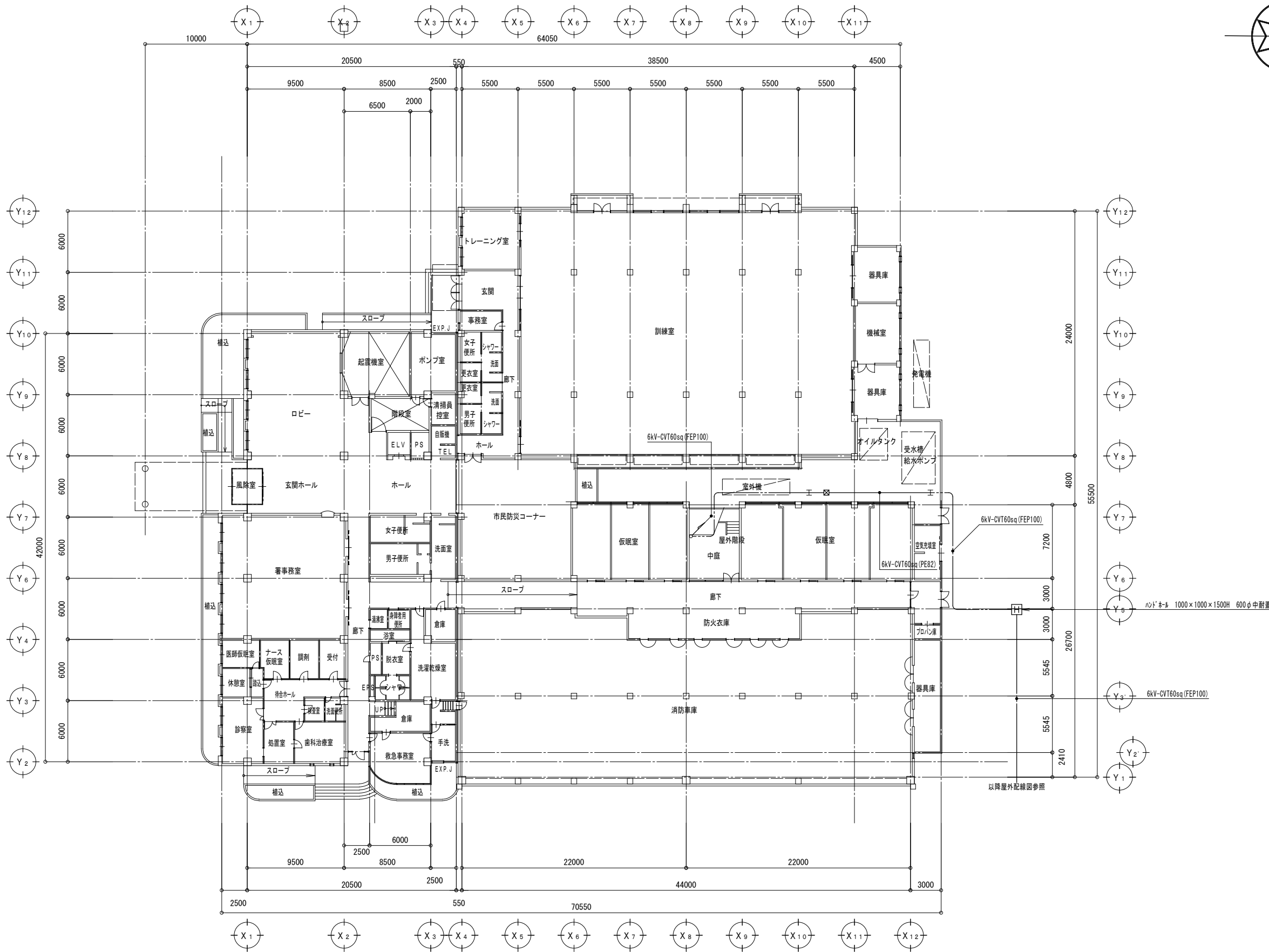
1階 平面図 (改修前) S=1/200
