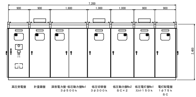
正面図 S=1/50 (姿図・寸法は参考とする)
