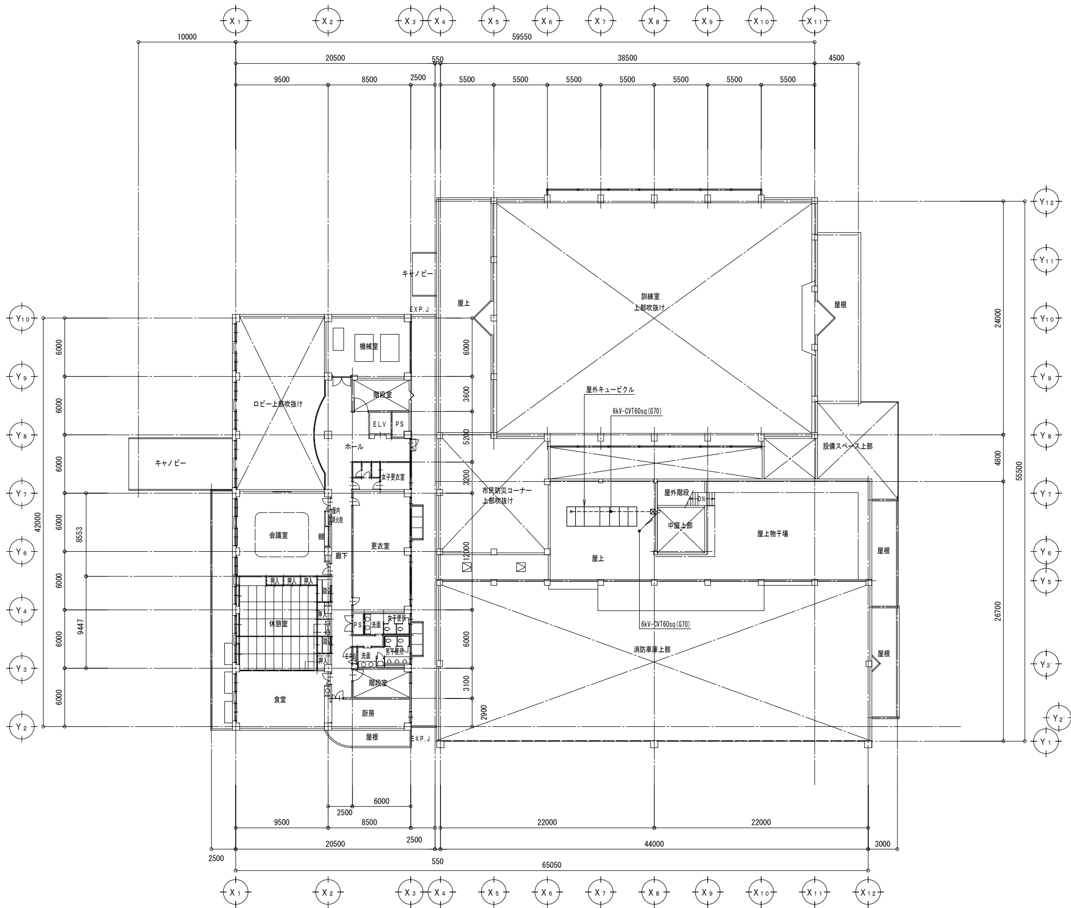
2階 平面図 (改修前) S=1/200
